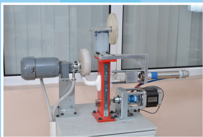
Uredjaj za testiranje izdržljivosti brave i kvake
